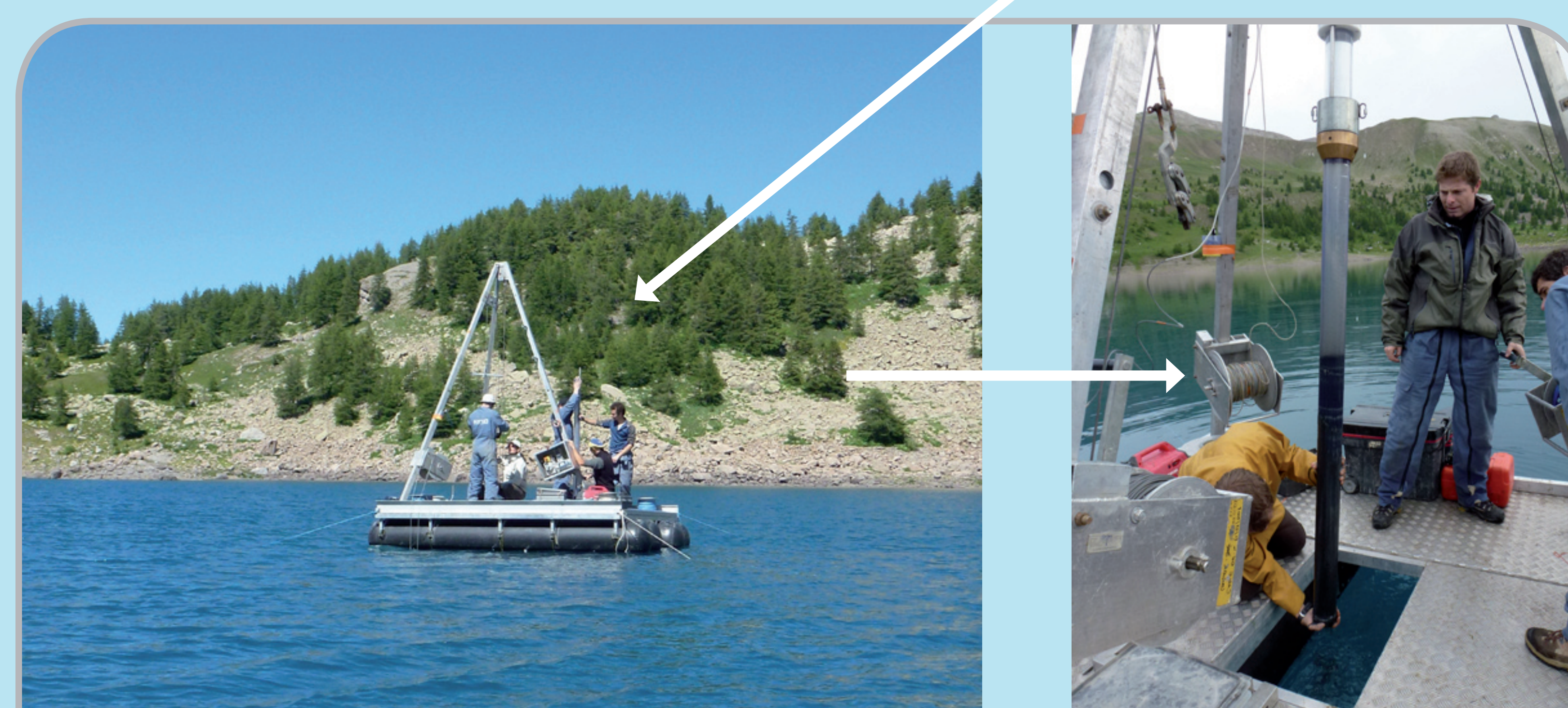
En Juillet 2011, un carottage est réalisé à 40 mètres de profondeur dans le lac d'Allos. Quinze mètres de sédiments sont prélevés. Une plate-forme flottante a permis de prélever les carottes de sédiments depuis la surface du lac.
